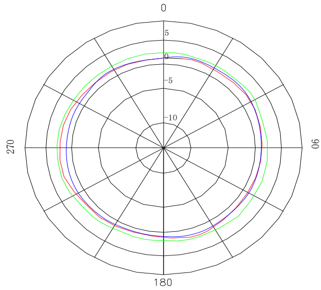
水平面方向图(2.4G天线) Horizontal Pattern
